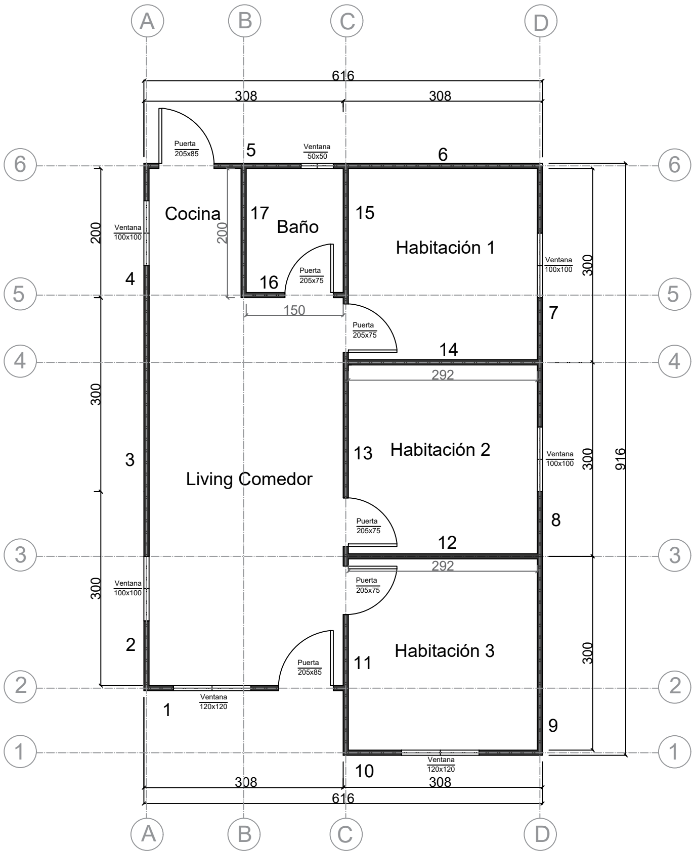
PLANTA NIVEL 1 - CASA 54 m 2
