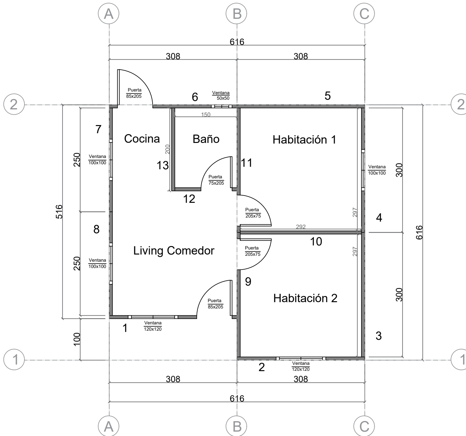
PLANTA NIVEL 1 - CASA 36 m 2
